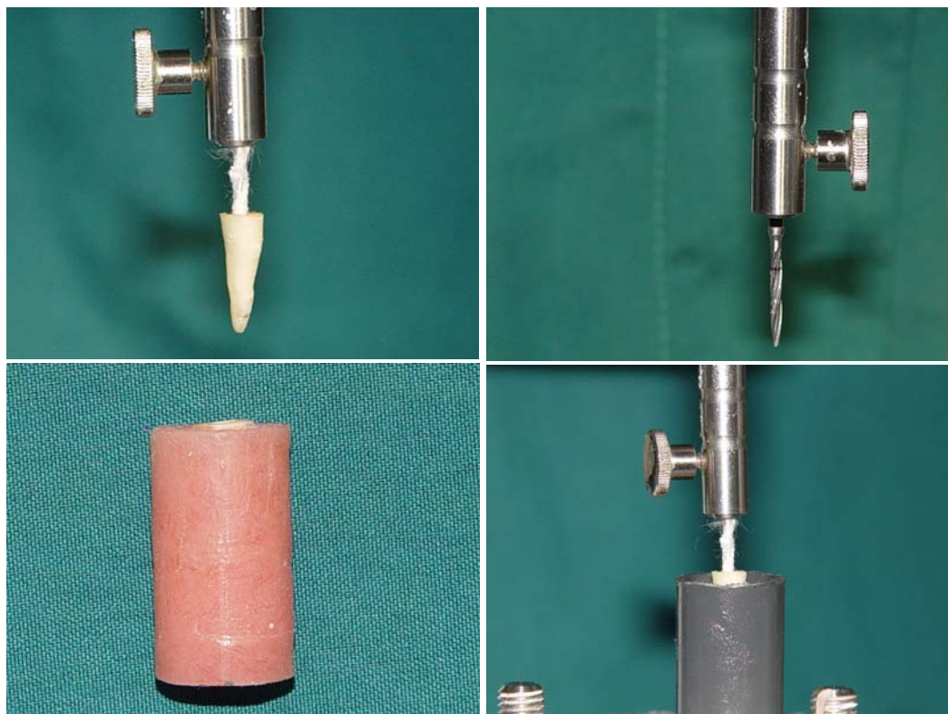
شکل ۲: قرار دادن نمونه‌ها در بلوک آکرلیکی توسط دستگاه سروپور
